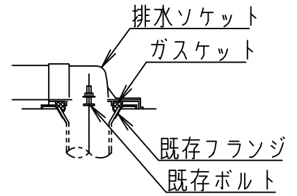
排水ソケットとフランジ部の固定
