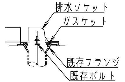
排水ソケットとフランジ部の固定
