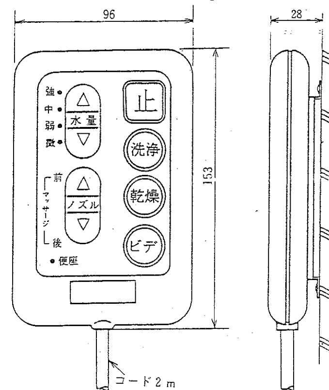
HC-201Dリモコン詳細
