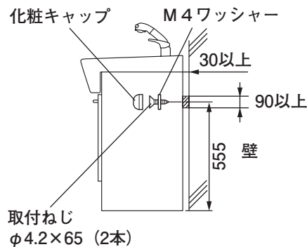
(補強材取付の場合)
