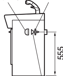
取付ねじ φ4.2×65（2本）
