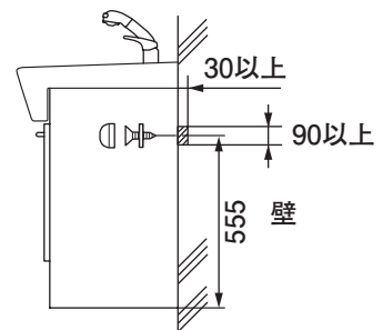
(補強材埋込みの場合)
