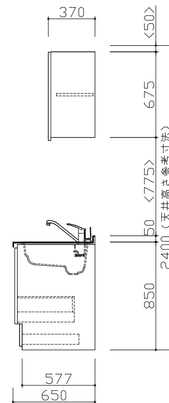
D側面図
