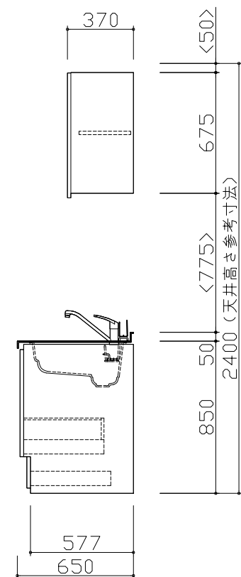
D側面図
