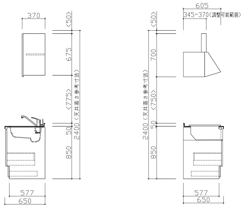
D側面図
