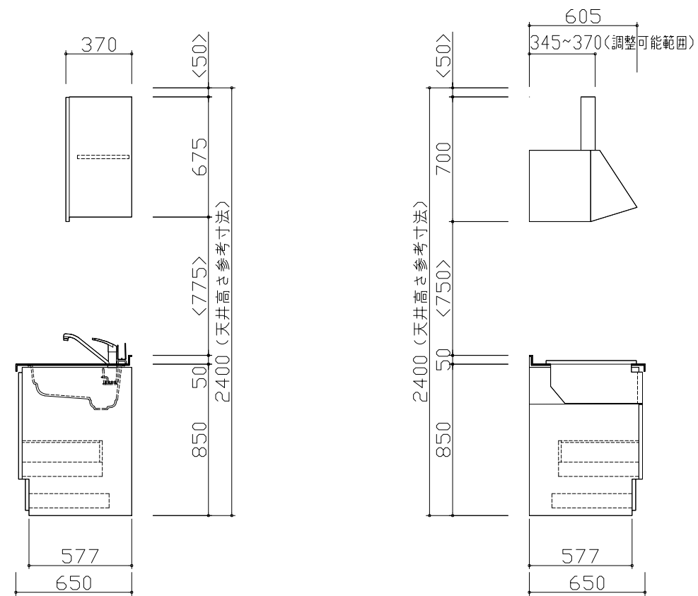
D側面図
