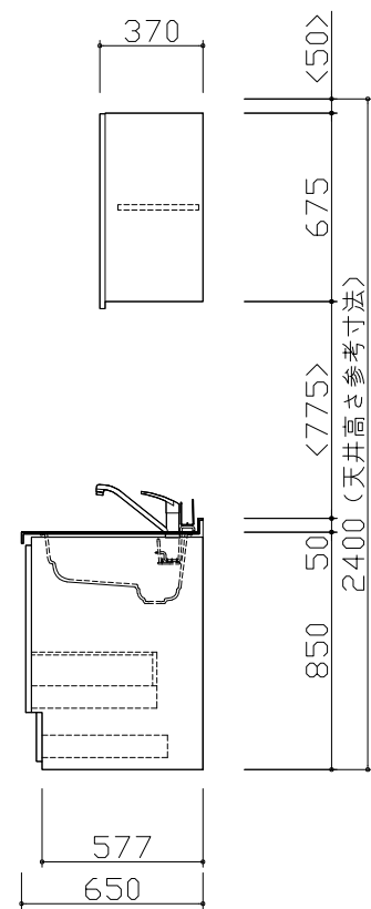
D側面図
