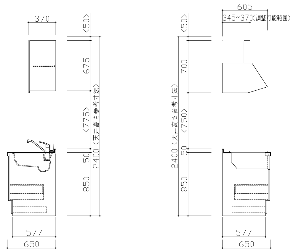
D側面図
