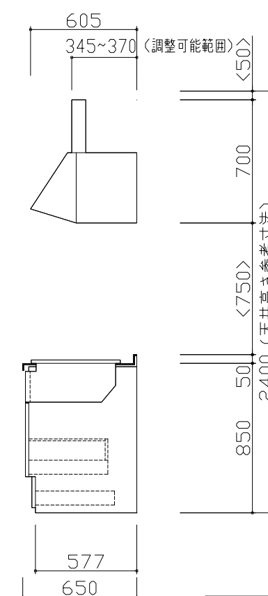
C背面図
