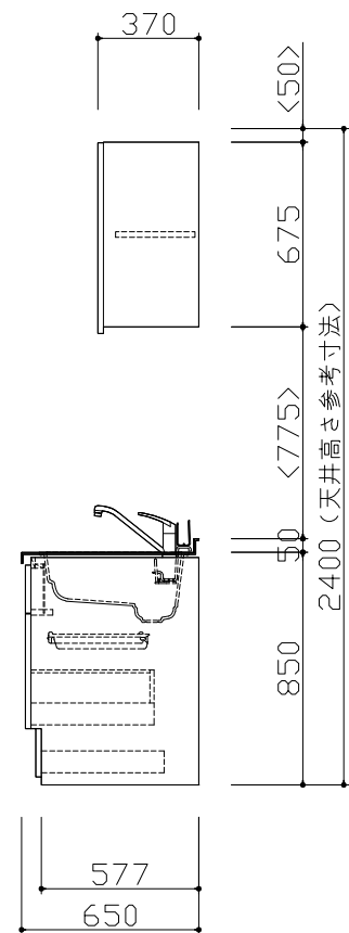
D側面図
