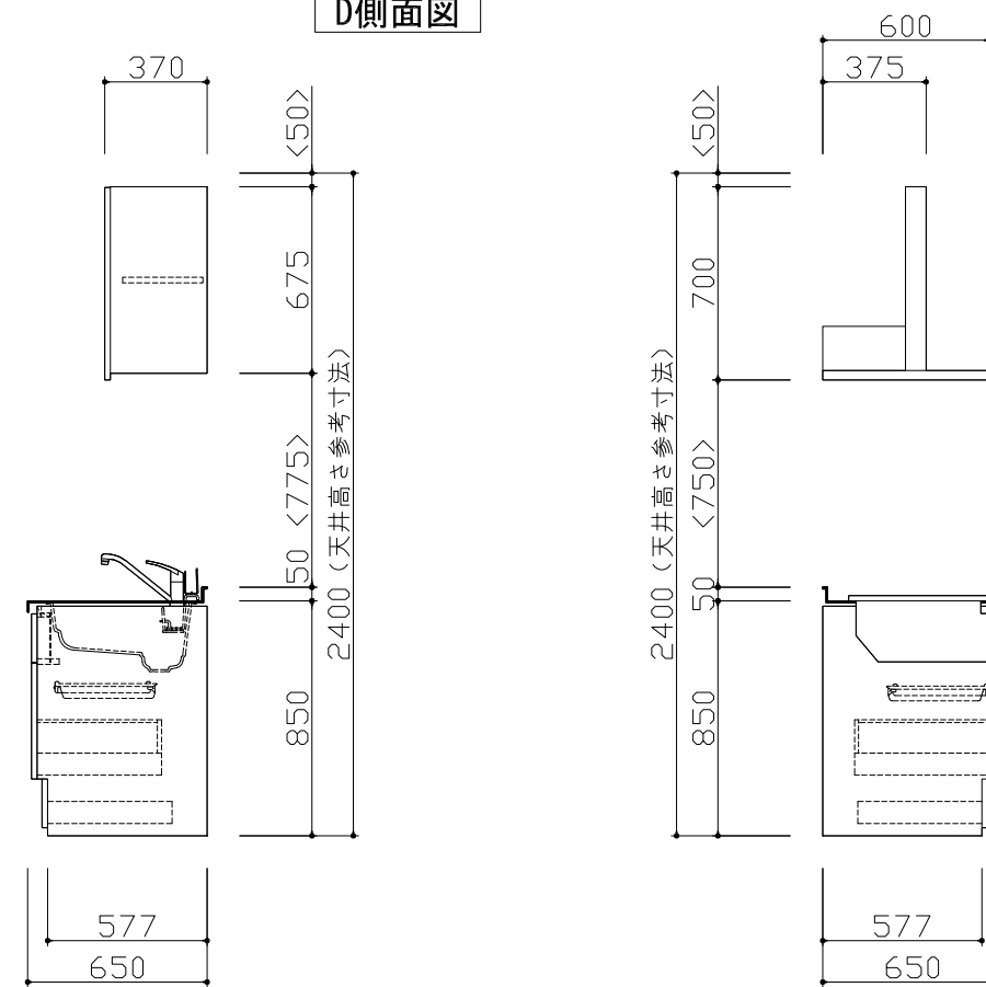
D側面図
