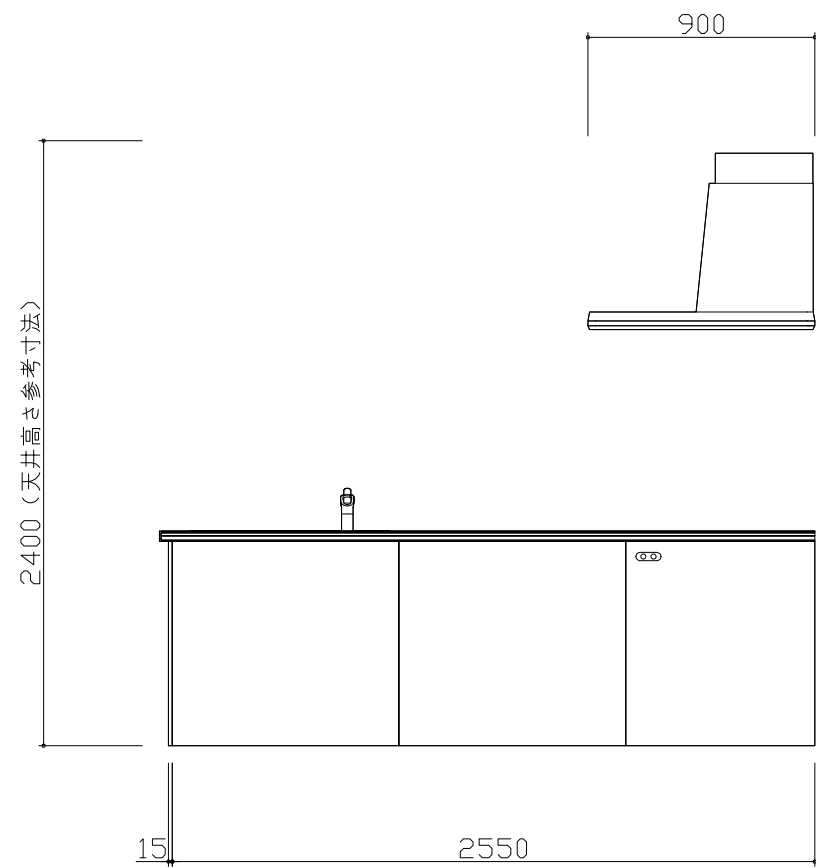
E立面图
