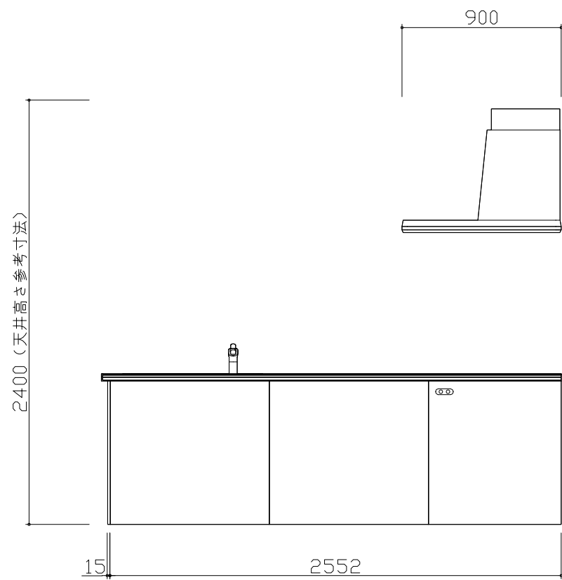
E立面图
