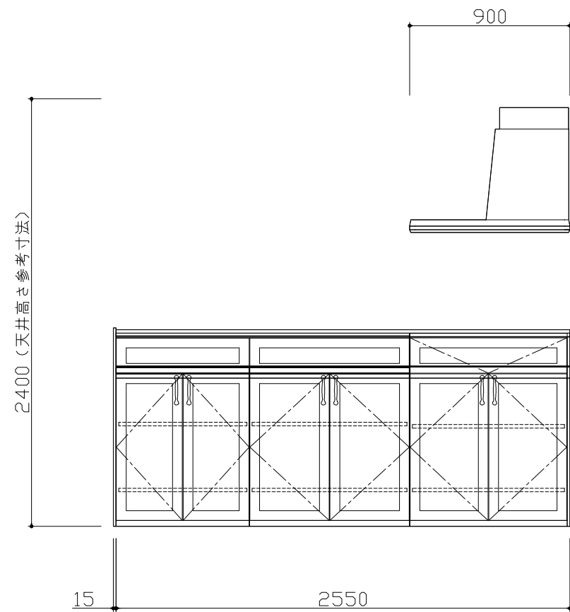
E立面图
