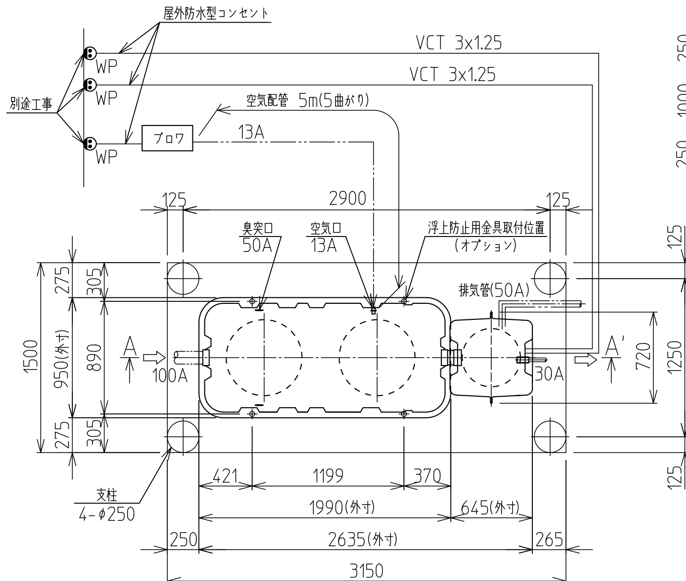
平面図
