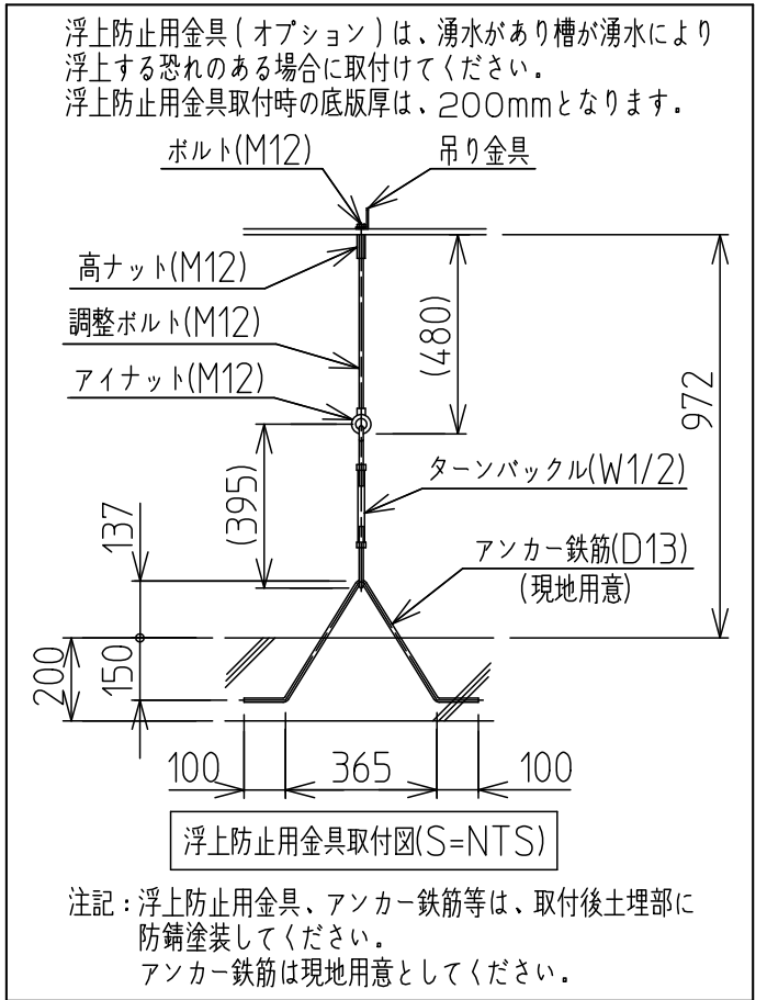
浮上防止用具(オプション例)
