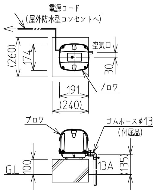
プロワ据付図(例) (尺度 N.T.S.)
