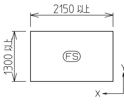
土間コンクリート(下)伏図
