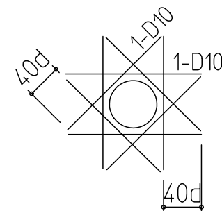
開口部補強筋
