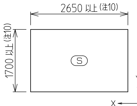
土間コンクリート(上)伏図
