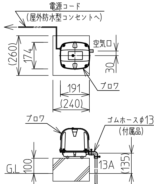
フロア据付図(例) (尺度 N.T.S)
