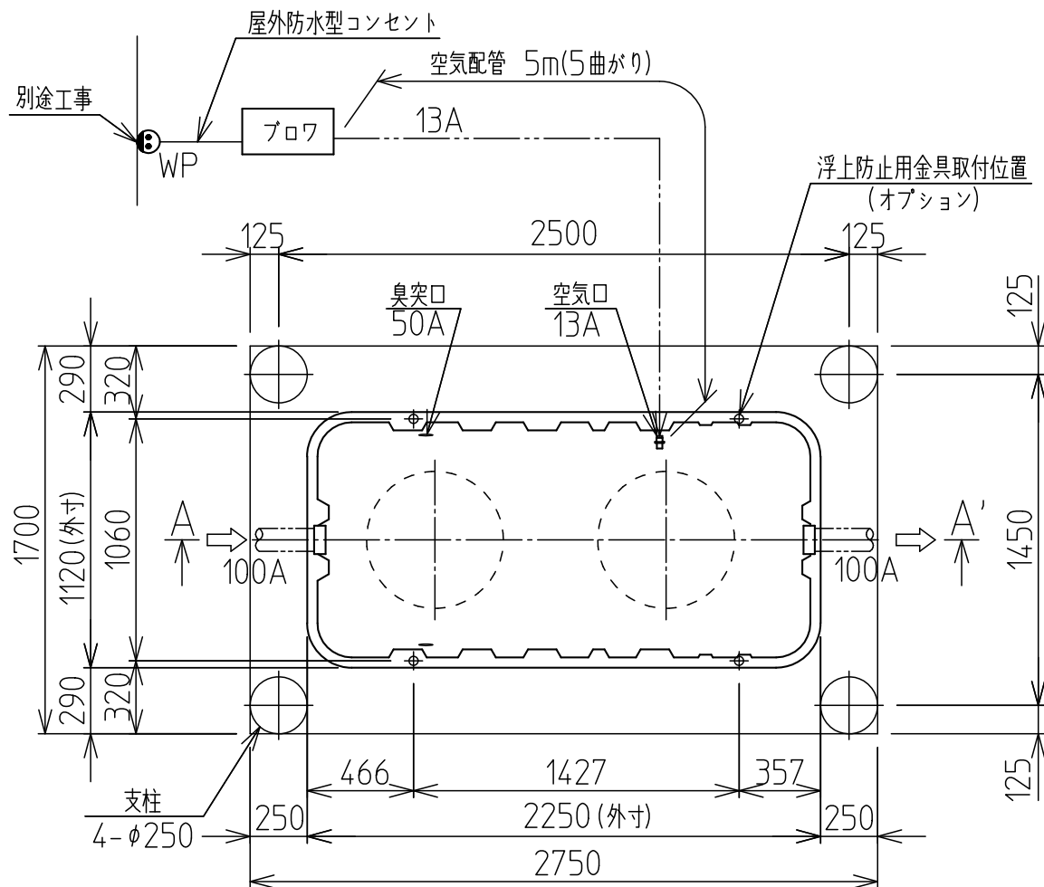
平面図
