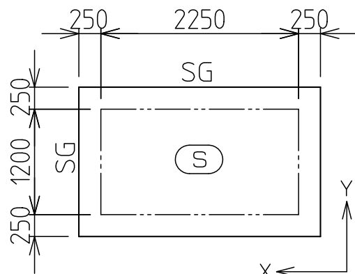
床スラブ伏図
