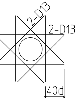
開口部補強筋
