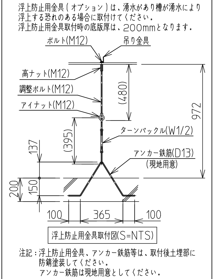
浮上防止用具(オプション例)
