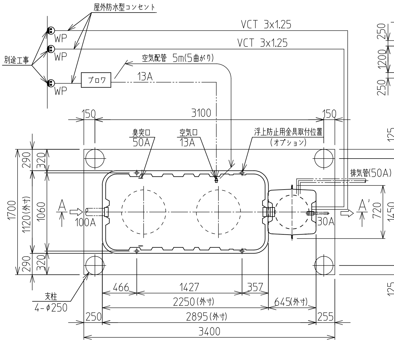
平面図
