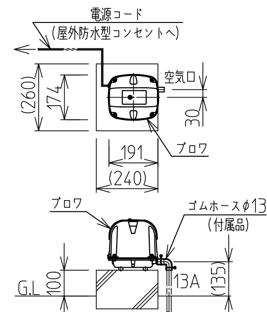
ブロー据付図(例) (尺度 N.T.S)
