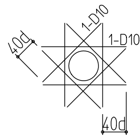
開 □ 部 補 強 筋
