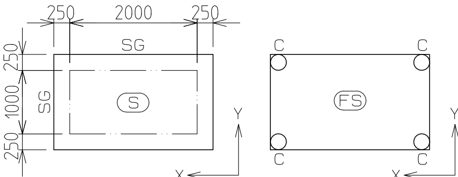
床スラブ伏図
