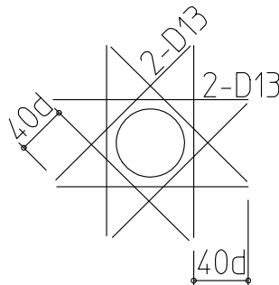
開口部補強筋
