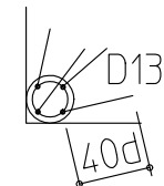
支柱配筋
