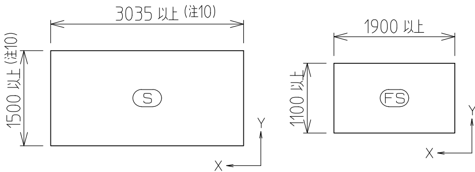
土間コンクリート(上)伏図
