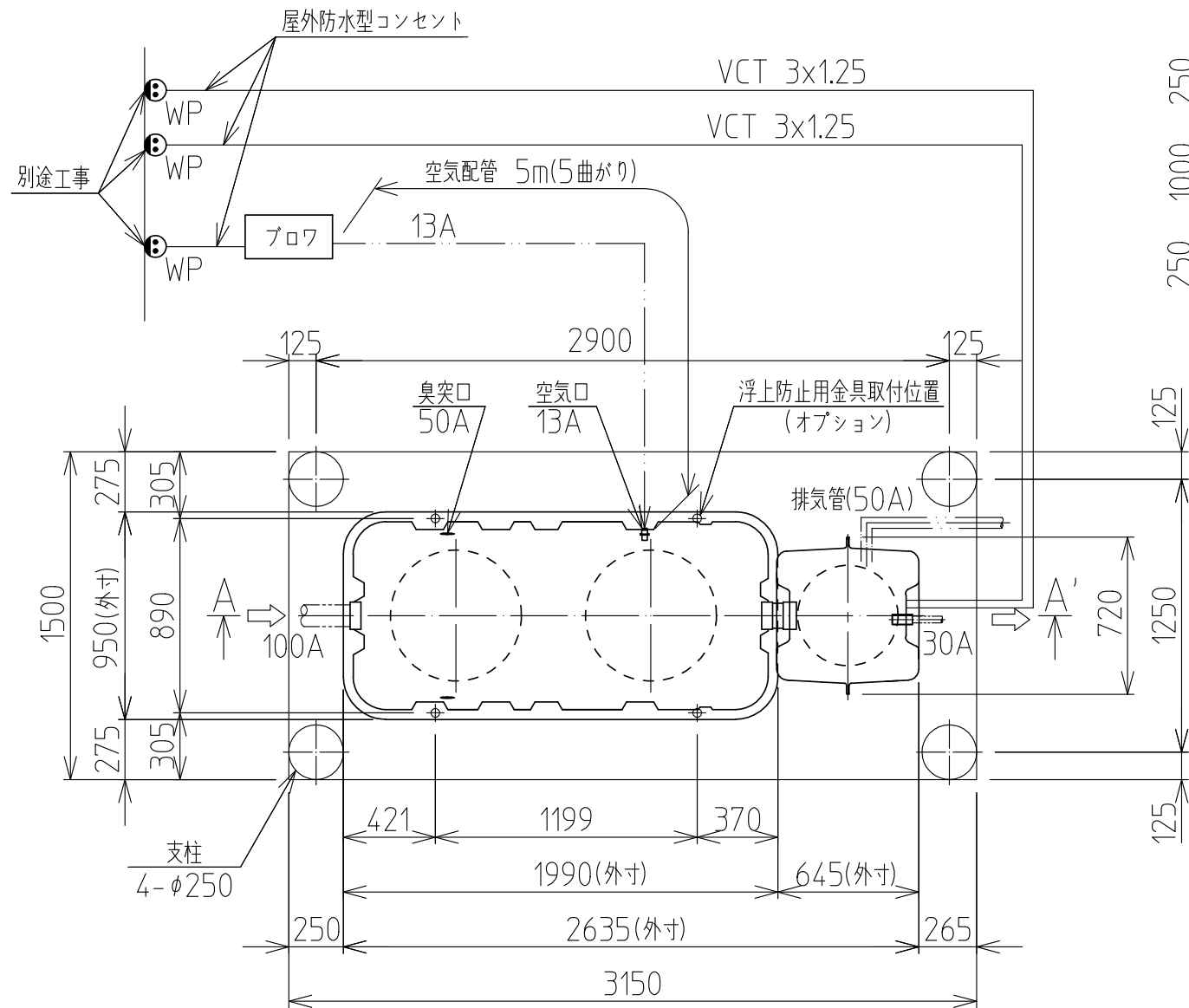
平面図
