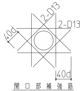
支柱配筋
