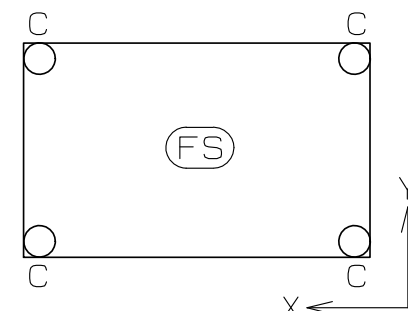
基礎スラブ伏図
