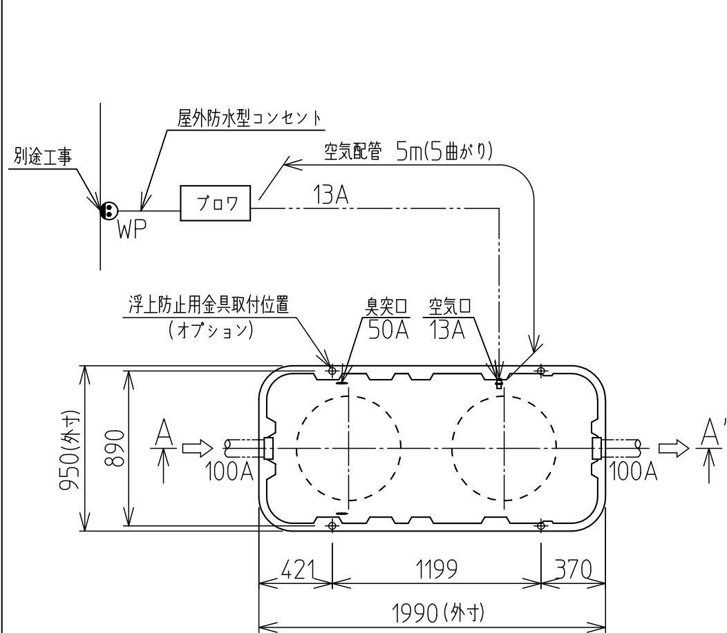
平面図
