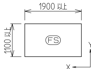
土間コンクリート(下)伏図
