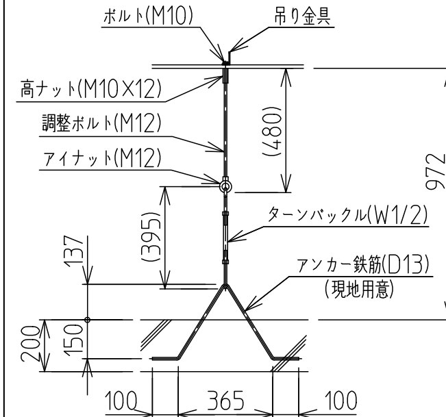
浮上防止用金具取付図(S=NTS)
