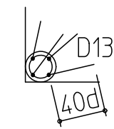
支柱配筋
