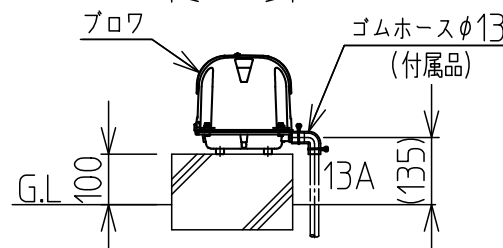
プロワ据付図(例) (尺度 N.T.S)
