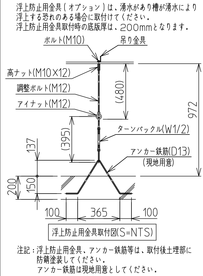
浮上防止用具(オプション例)
