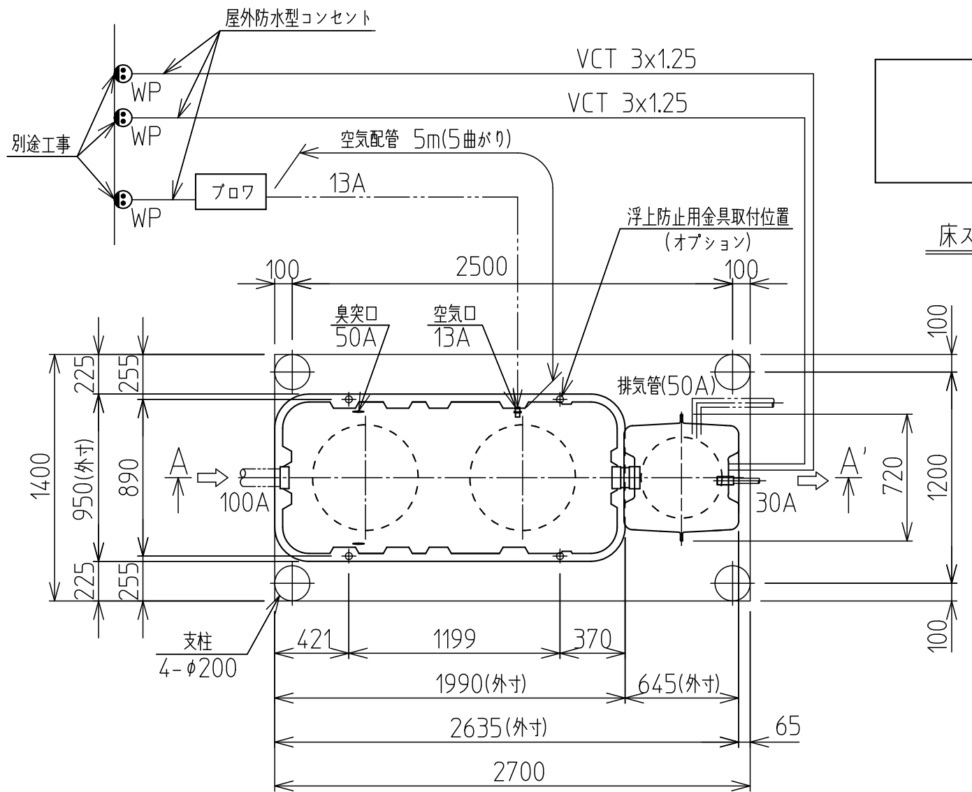
平面図
