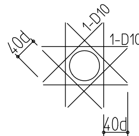
開 □ 部 補 強 筋
