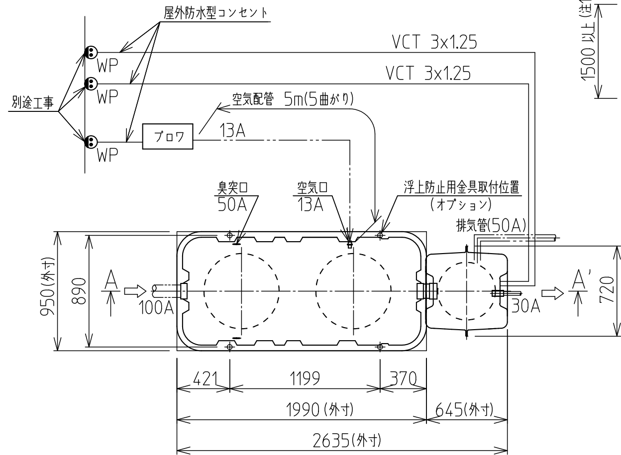
平面图
