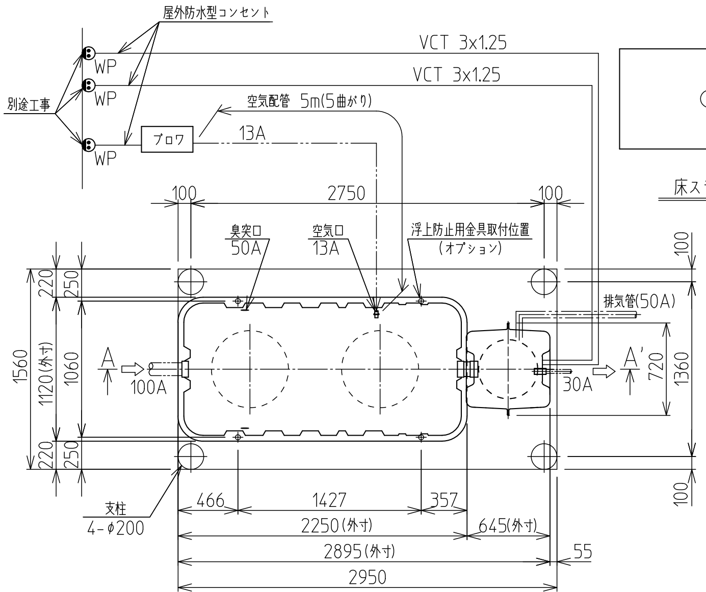
平面図
