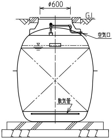
B-B'断面図
