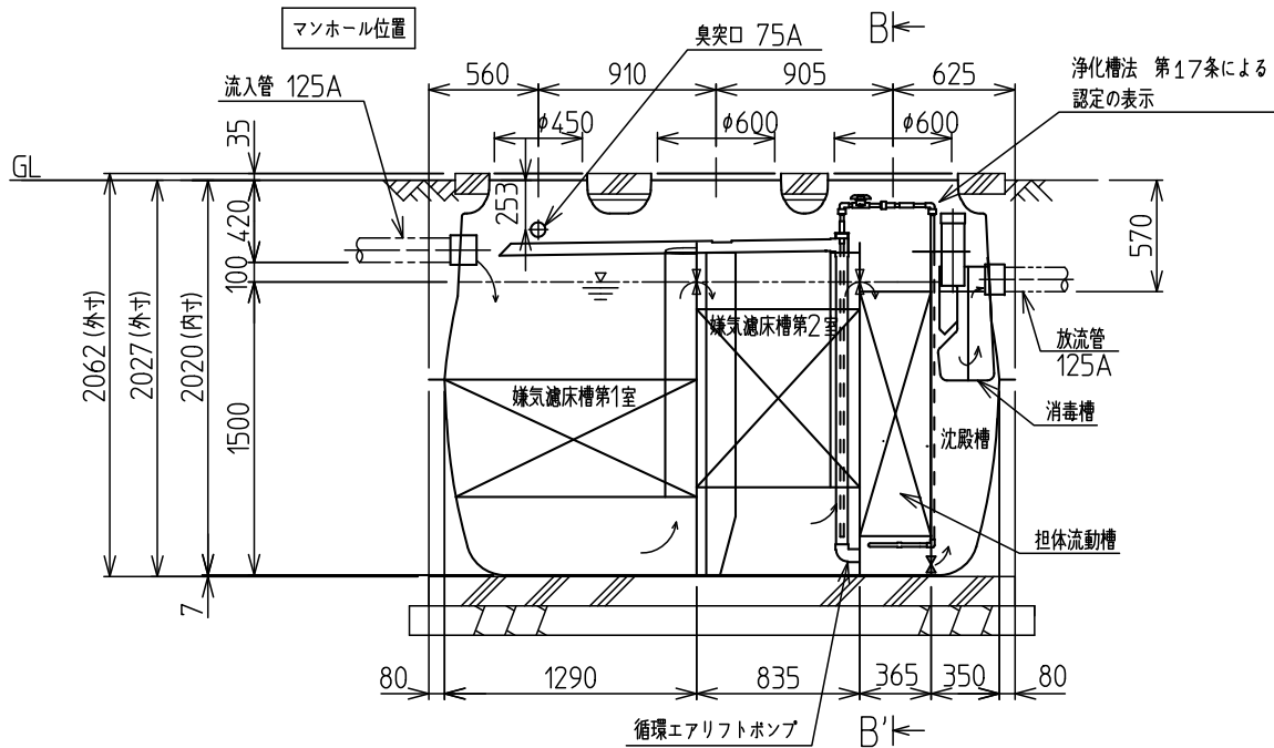
A-A'断面図
