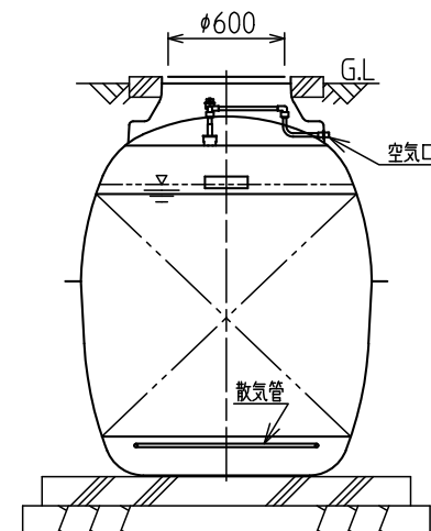
B-B' 断面图
