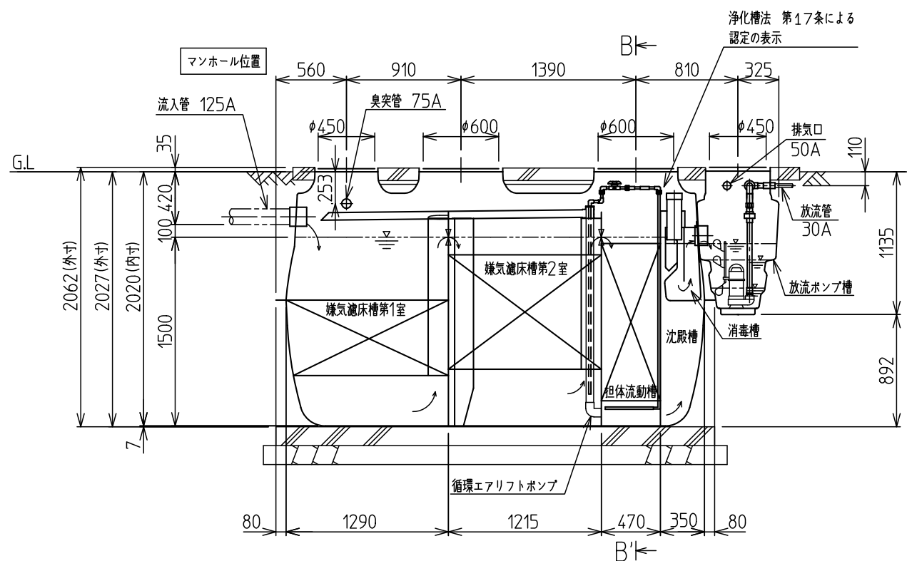
A-A'断面图
