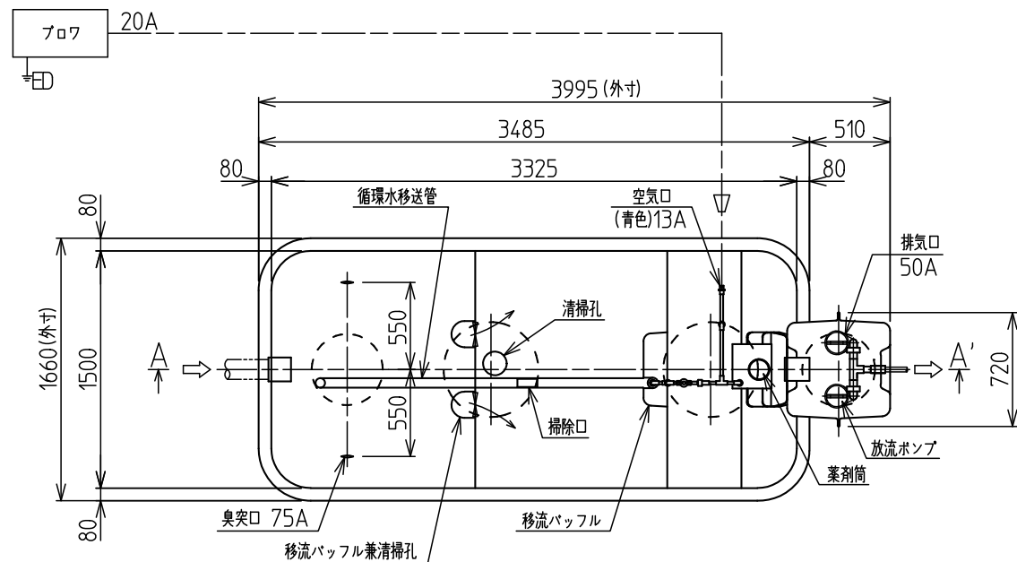
平面图
