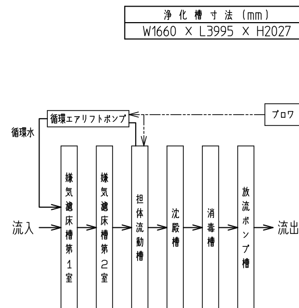
フローシート
