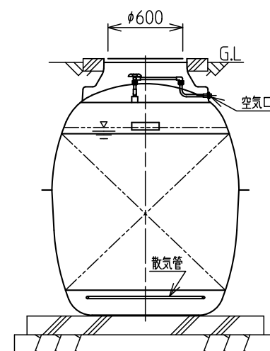
B-B'断面图
