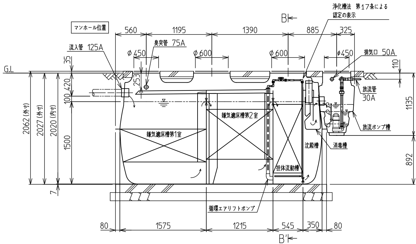
A-A'断面図
