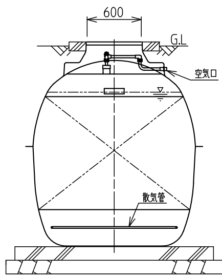
B-B'断面図
