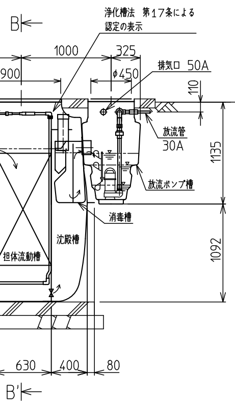
A-A'断面図
