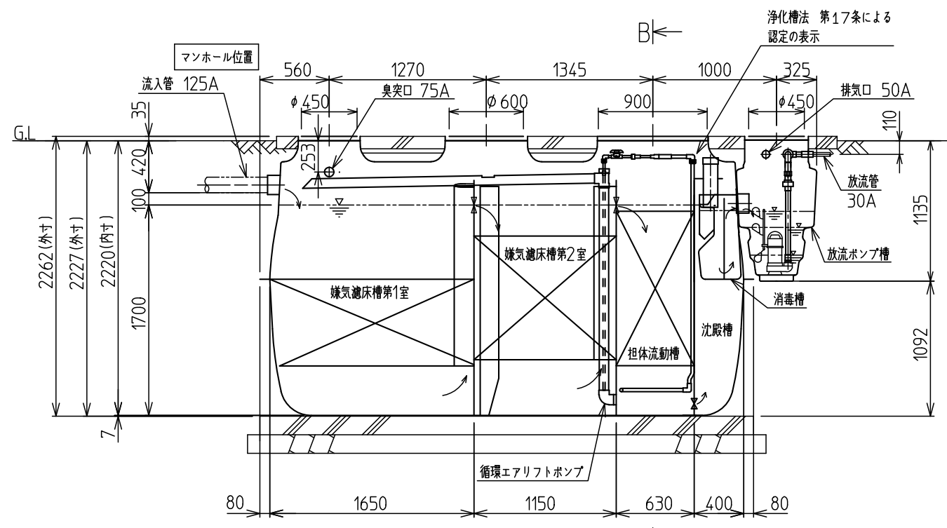
A-A'断面図
