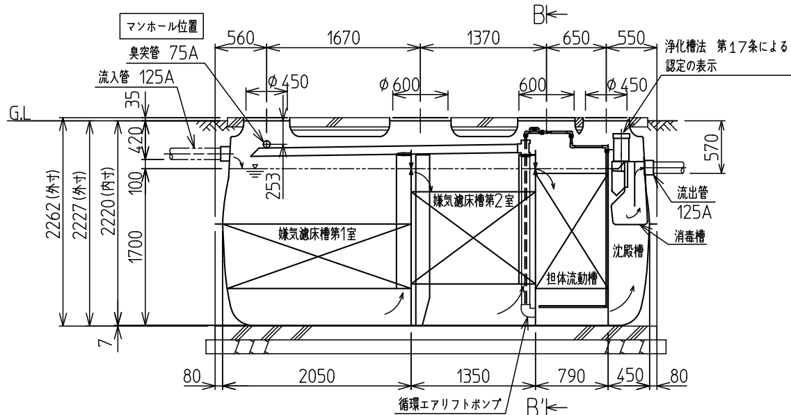
A-A'断面図
