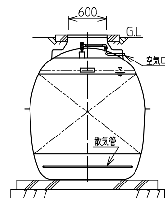
B-B'断面图
