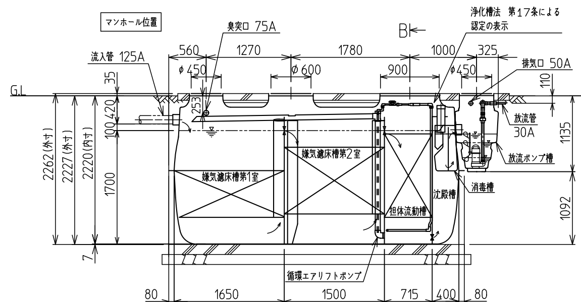
A-A' 断面図
