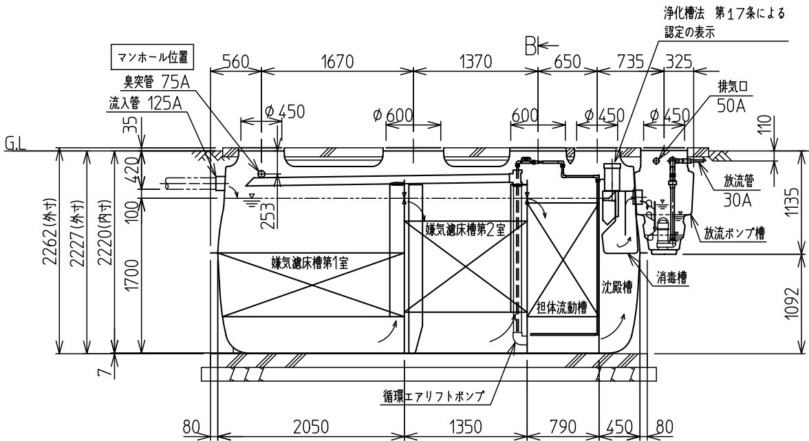
A-A'断面図
