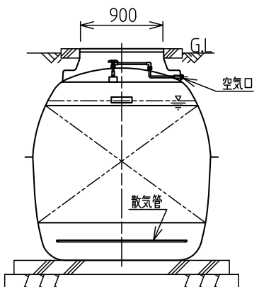
B-B'断面図
