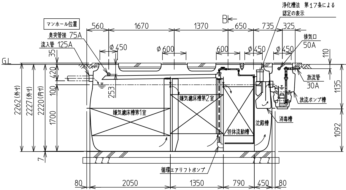
A-A'断面図
