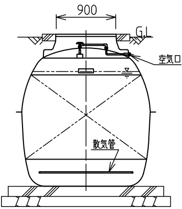
B-B'断面図
