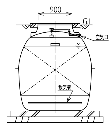
B-B'断面図
