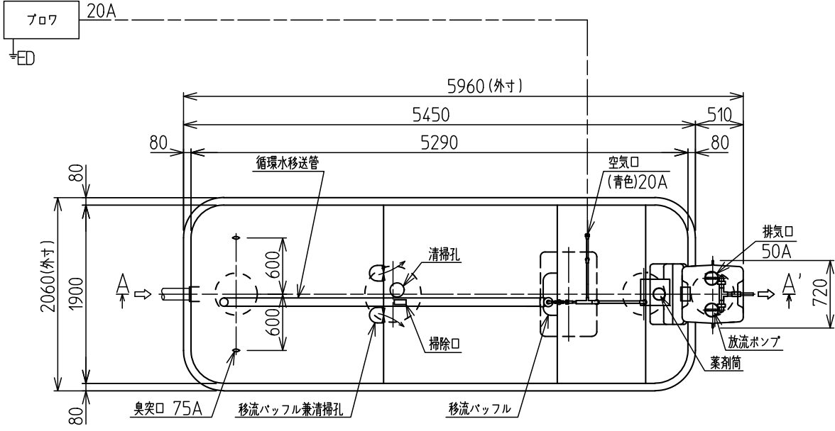
平面図
