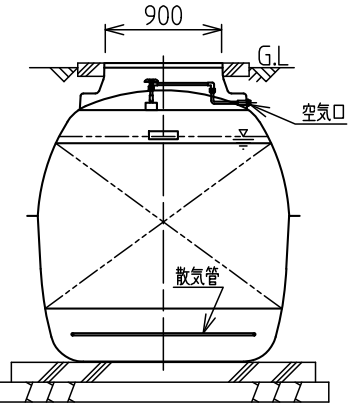
B-B'断面図
