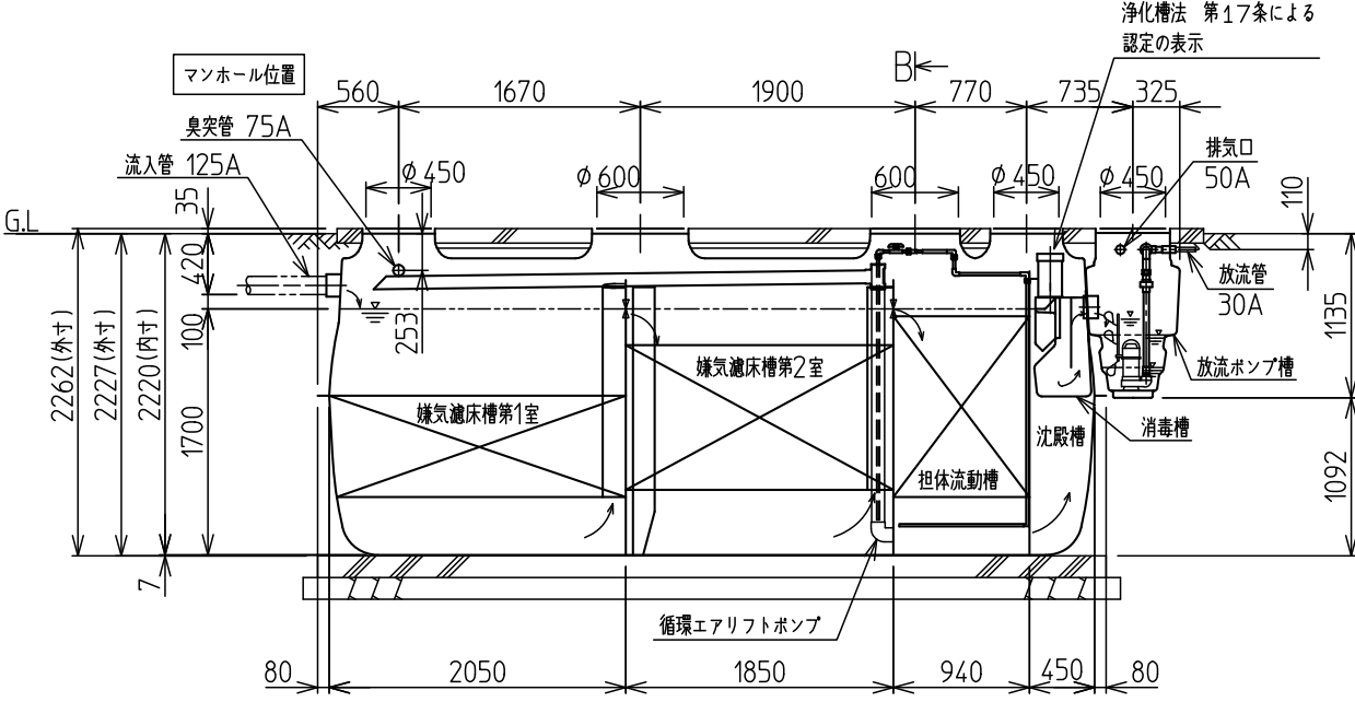
A-A'断面図
