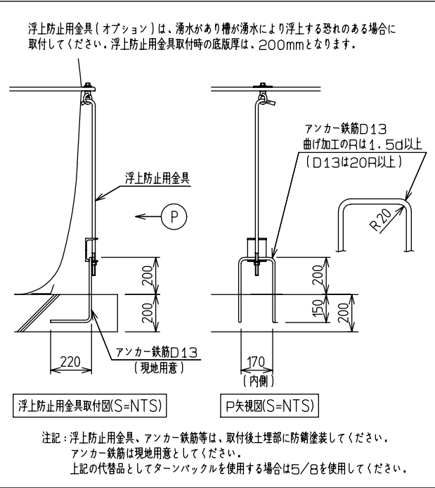
浮上防止用具 (オプション例)
