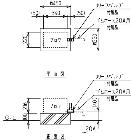
フロワ据付図(例) (尺度 N.T.S)
