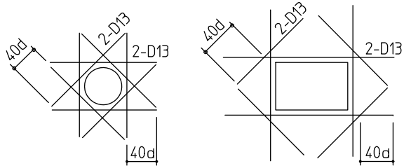
浮上防止用具(オプション例)
