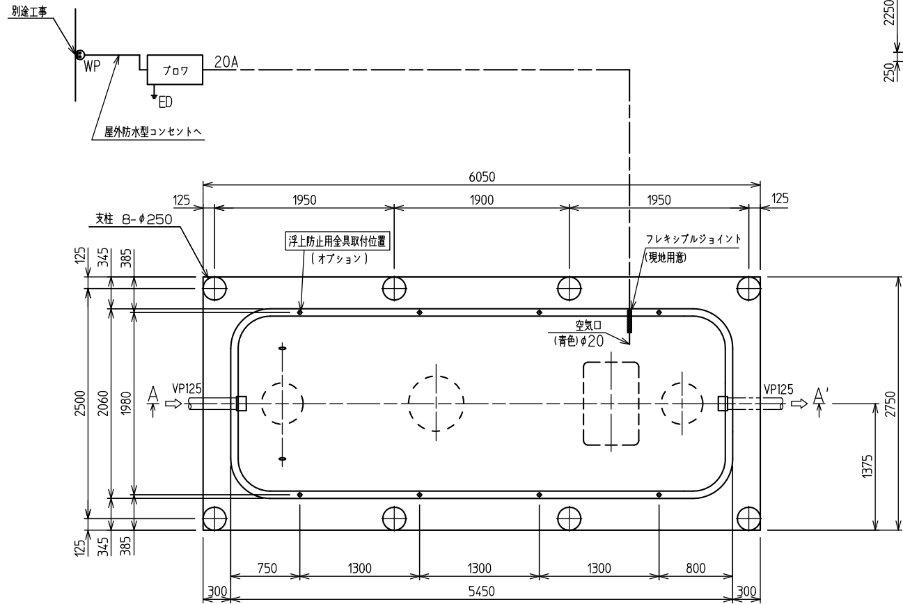
平面図
