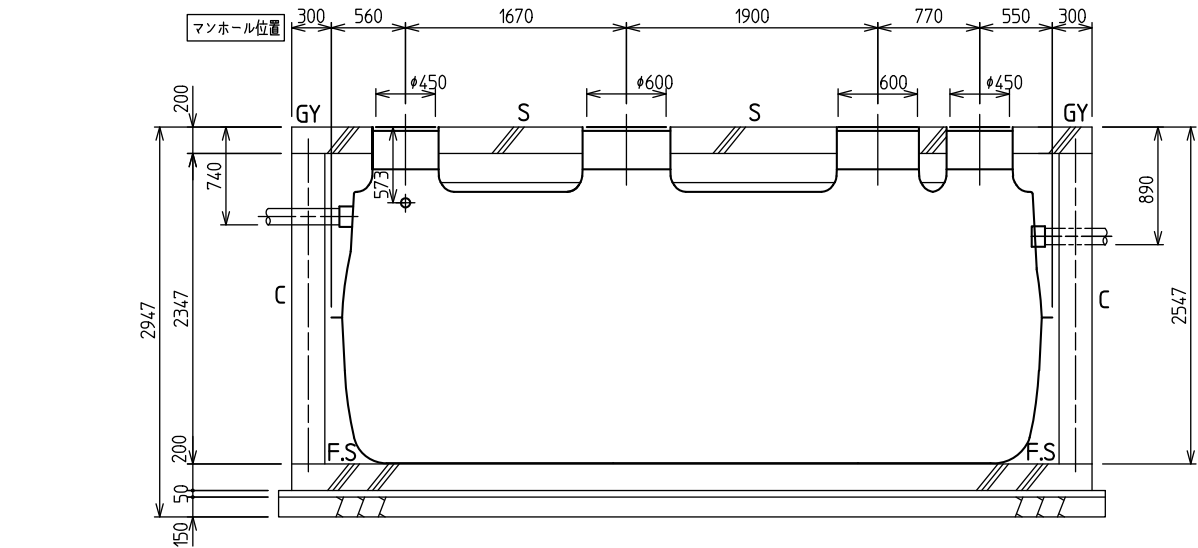
A-A'断面図
