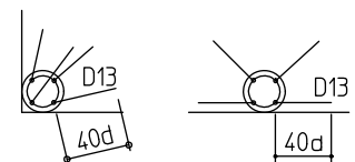
支 柱 配 筋
