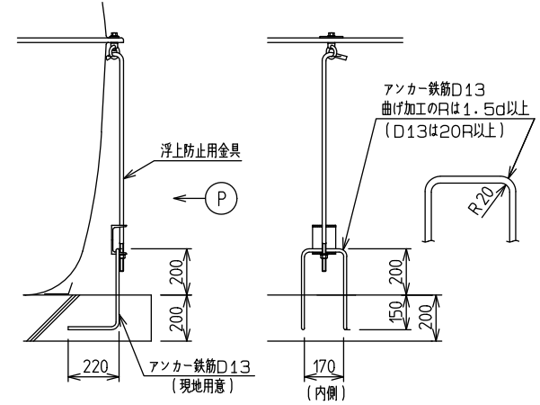
浮上防止用金具取付図(S=NTS)
