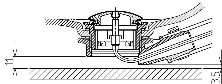
排水口部詳細図
